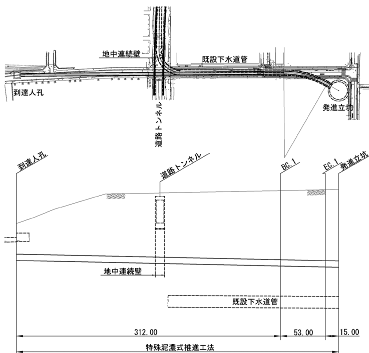
図-1 設計概要
